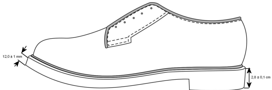
ΣΧΕΔΙΟ 12 ΠΑΧΟΣ ΣΟΛΑΣ - ΤΑΚΟΥΝΙΟΥ
